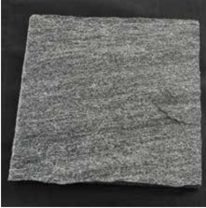
32493 1080.00/t Calanca bruchroh 4 – 6 x 30 – 50 x freie Längen Kanten zum Teil gesägt oder bruchroh
